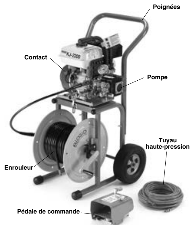
Figure 1 – Dégorgoir haute-pressure KJ-2200
