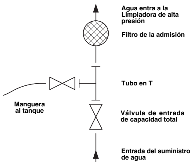
Figura 9 – Conexiones al emplearse un tanque de agua como suministro
