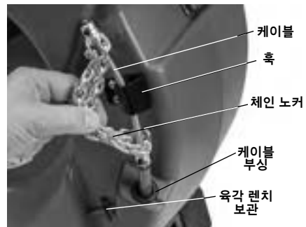
그림 1C – 케이블 끝/체인 노커
