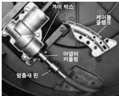
그림 15 – 열려 있는 드레인 클리너 하우징
