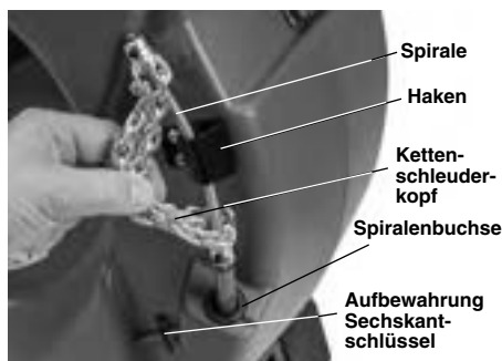
Abbildung 1C – Spiralenende/ Kettenschleuderkopf
