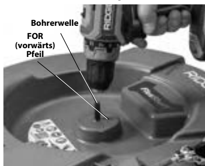
Abbildung 4 – Befestigung des Bohrers an der Bohrerwelle
