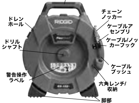
図 1A – RIDGID® FlexShaft（フレックスシャフト）排水管清掃機
