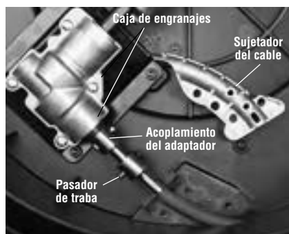
Figura 15 – Apertura del alojamiento de la limpiadora de desagües
