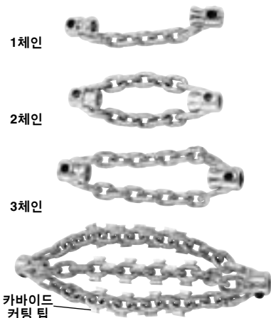
그림 8 - 체인 노커
