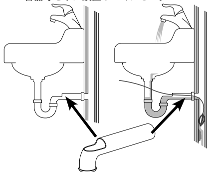
図 3 - 壁パイプの設置
