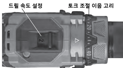
그림 6 - 드릴 설정
