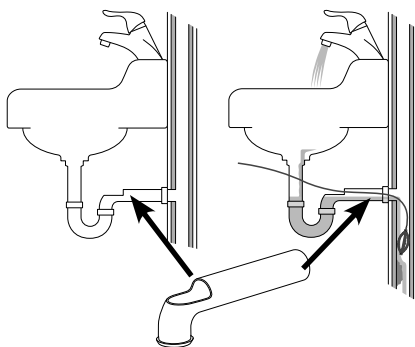
그림 3 - 벽 파이프 설치
