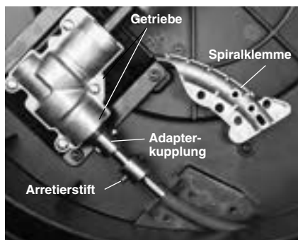
Abbildung 15 – Geöffnetes Gehäuse der Abflussreinigungsmaschine
